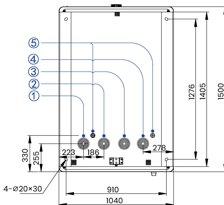
Монтажні отвори в нижній пластині (вид зверху) (одиниця виміру: мм)
