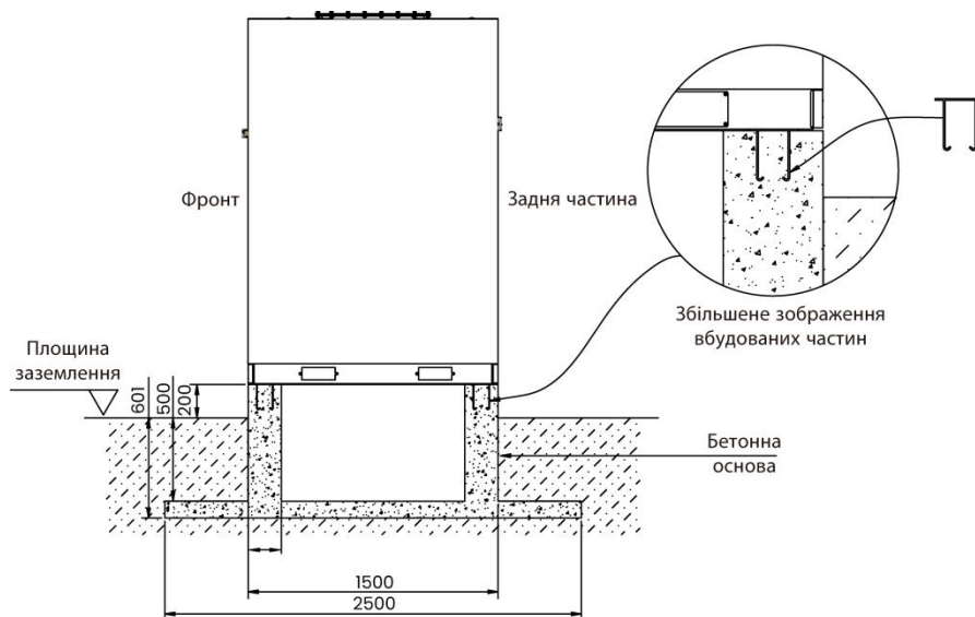
Секція монтажної основи (вид збоку) (одиниця виміру: мм)
