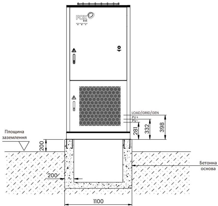
Секція монтажної основи (вид спереду) (одиниця виміру: мм)
