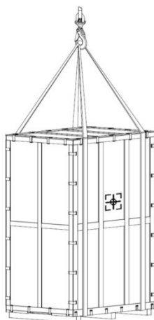
Принципова схема підйому та переміщення з упаковкою
