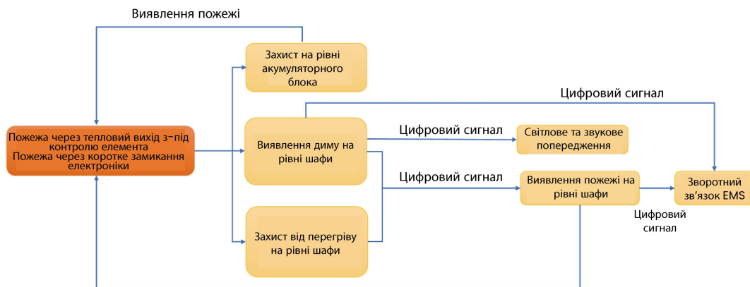
Логіка керування системою пожежі
