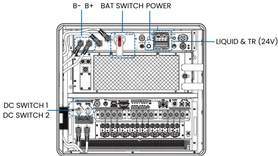
Внутрішня схема нижньої коробки корпусу
